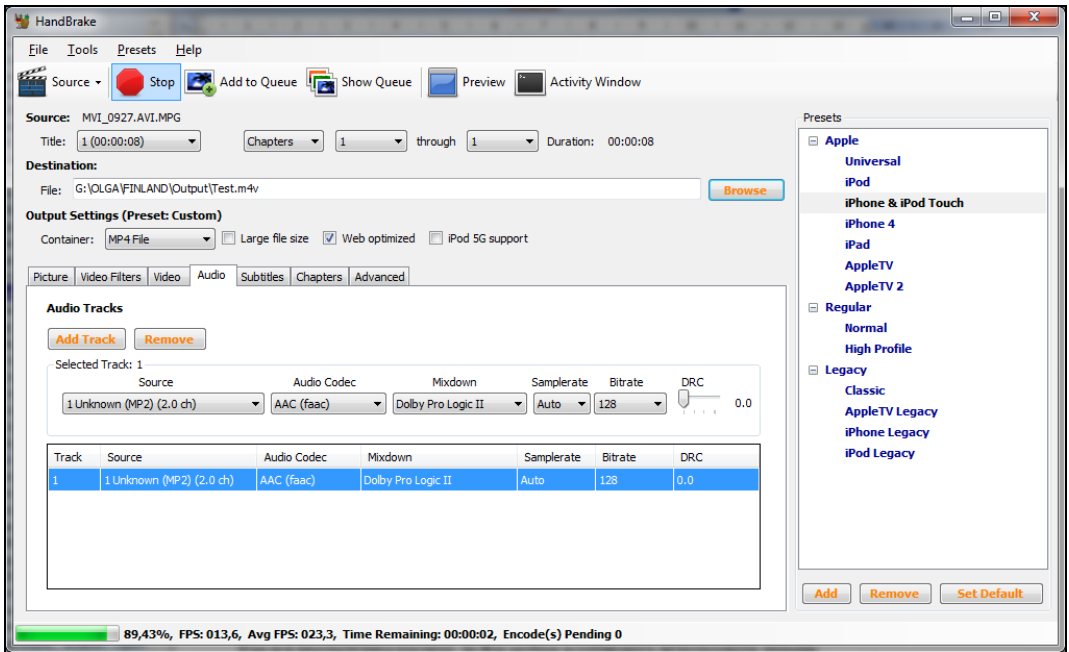
Рис. 5.28. Наберитесь терпения!
