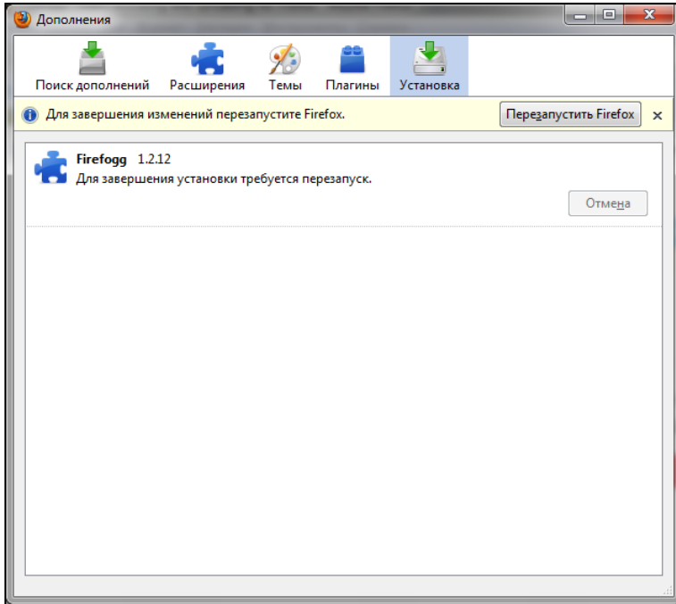
Рис. 5.12. Перезапуск Firefox
