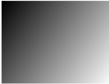
Рис. 4.12. Диагональный градиент
