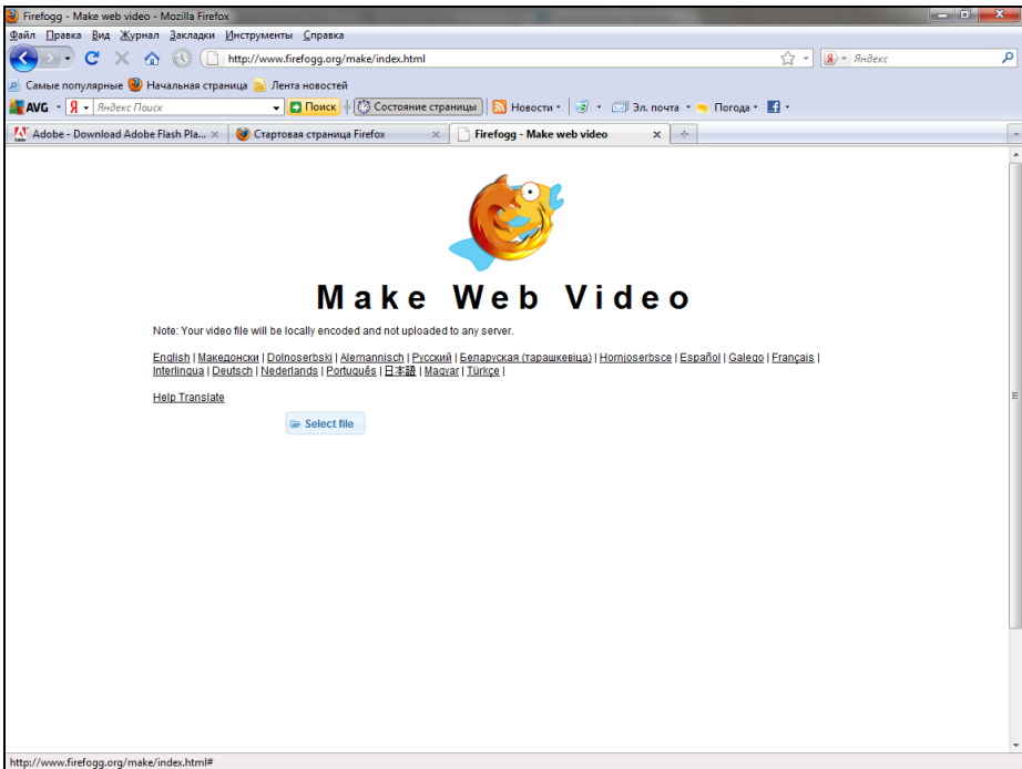
Рис. 5.15. Выбор видеофайла
