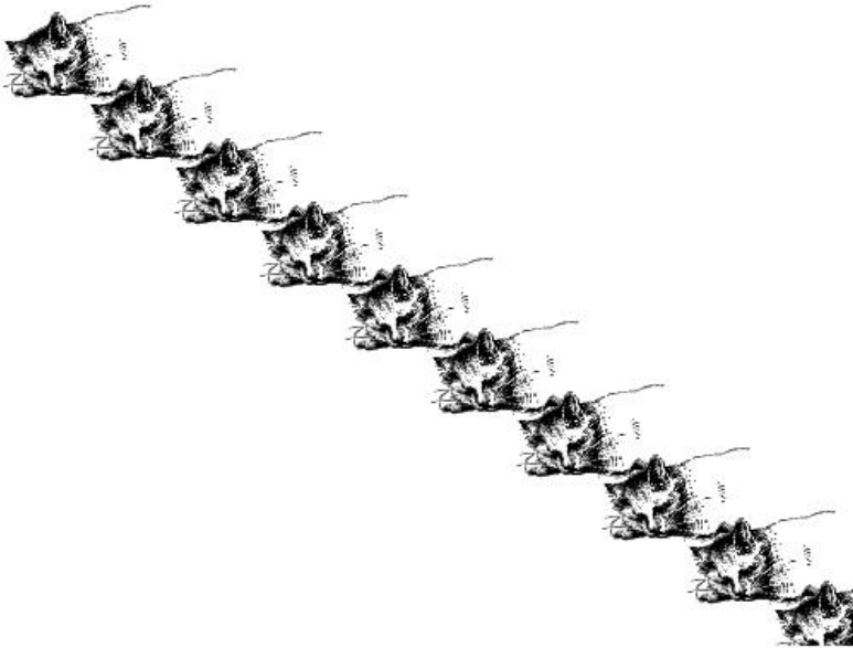
Рис. 4.15. Клонирование кошек!
